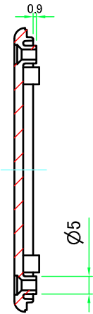
C-C ( 1 : 1.5 )
